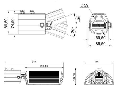
Габаритный чертеж
