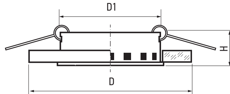
Рис. 1. Светильник PGX53d
