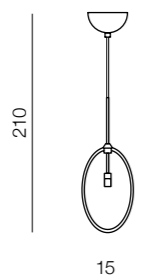
Diana 1 AZ2150 G9 1x MAX 40W glass/metal
