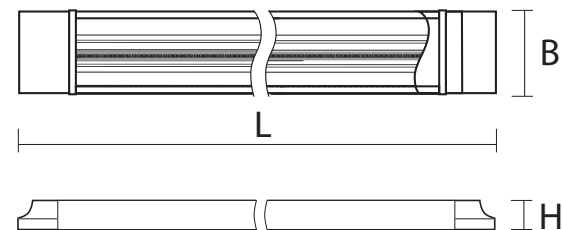
Рис. 1 Светильник РР0-04
